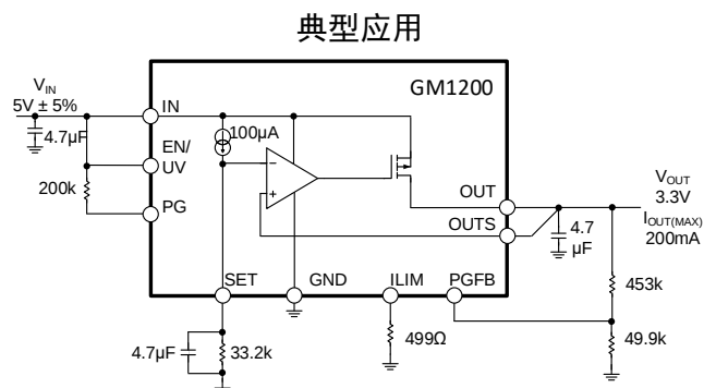
图 1 典型应用
