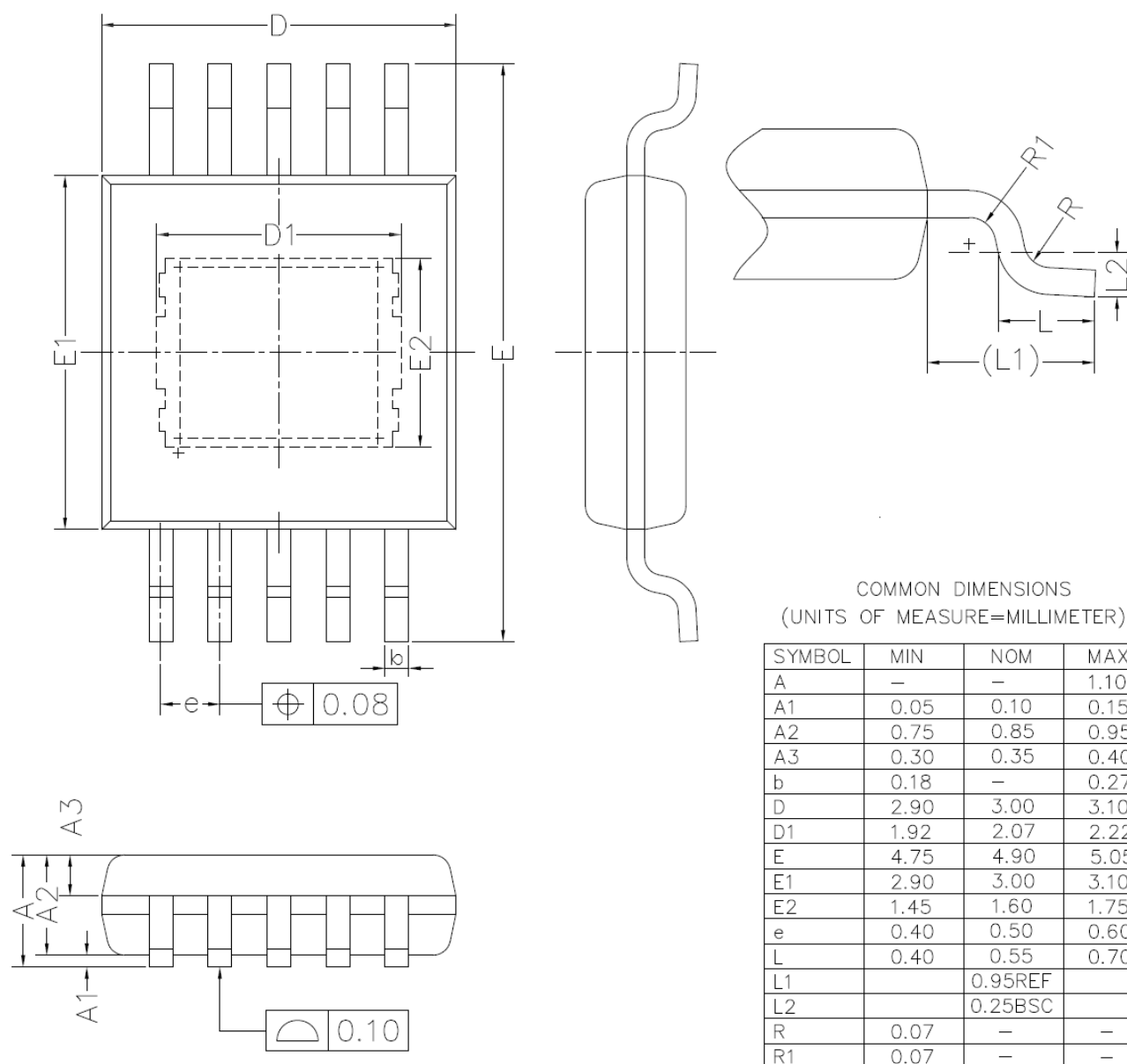
图 24 MSOP 封装
