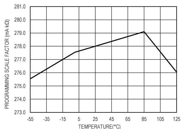
图 15. 输出限流值编程因子
