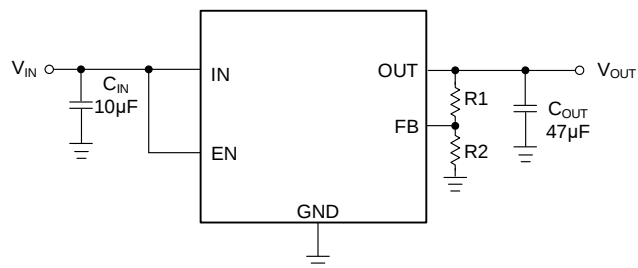
图 1 典型应用
