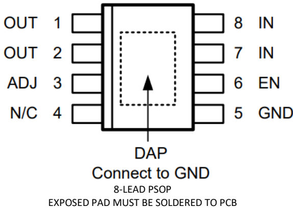
图 2 引脚配置
