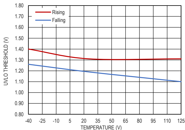
图 9. UVLO 阈值
