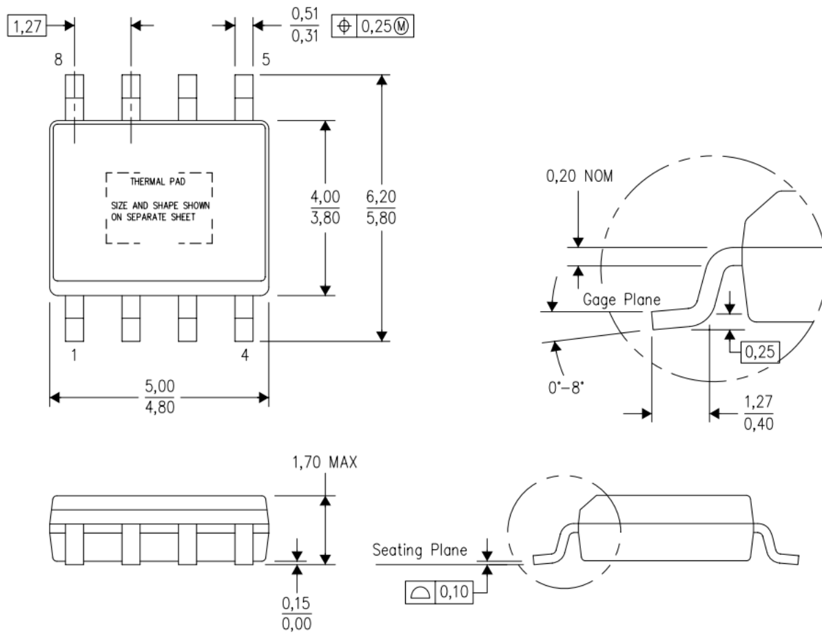
图 18. 8 引脚 PSOP
