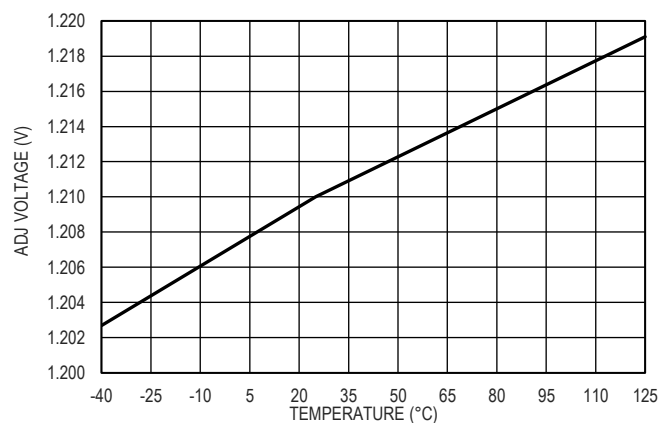
图 11. ADJ 引脚电压精度
