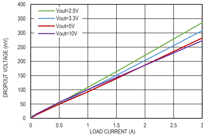
图 4. 压差电压和负载电流的关系
