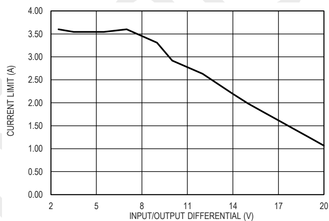
图 13. 输出限流值和输入输出压差的关系
