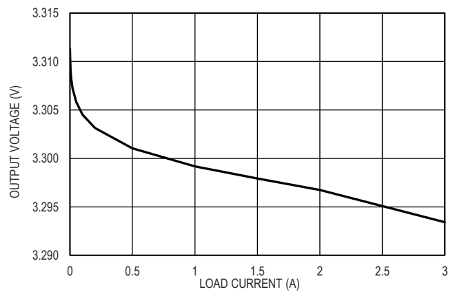
图 9. 3.3V 输出电压和负载电流的关系
