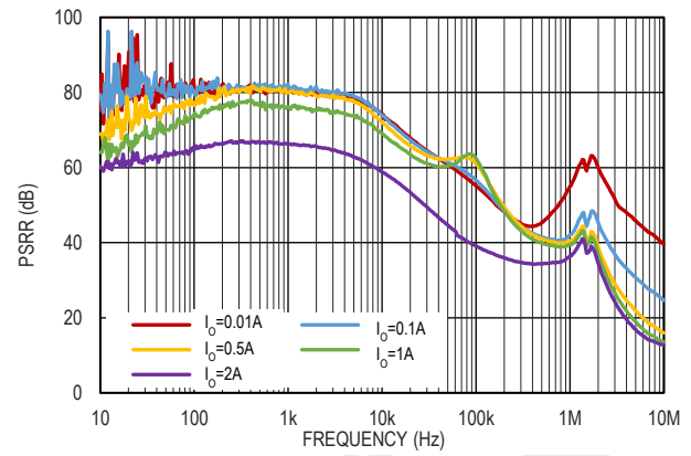
图 17. 电源电压纹波抑制比, V_{IN}=5V , V_{OUT}=3.3V
