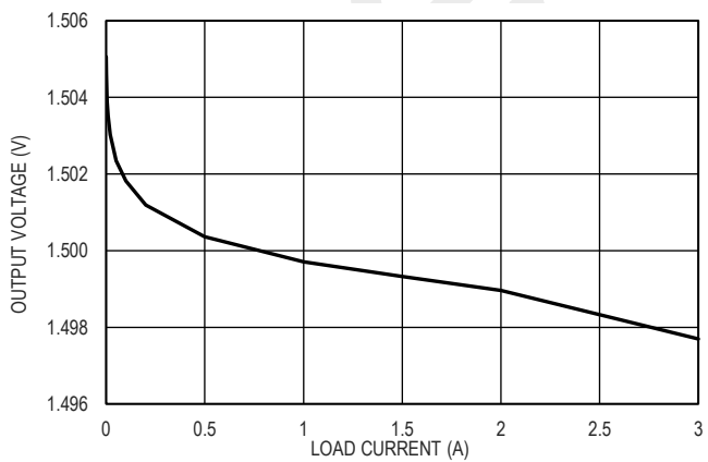
图 8. 1.5V 输出电压和负载电流的关系
