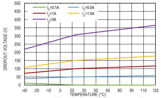
图 5. 压差电压和温度的关系
