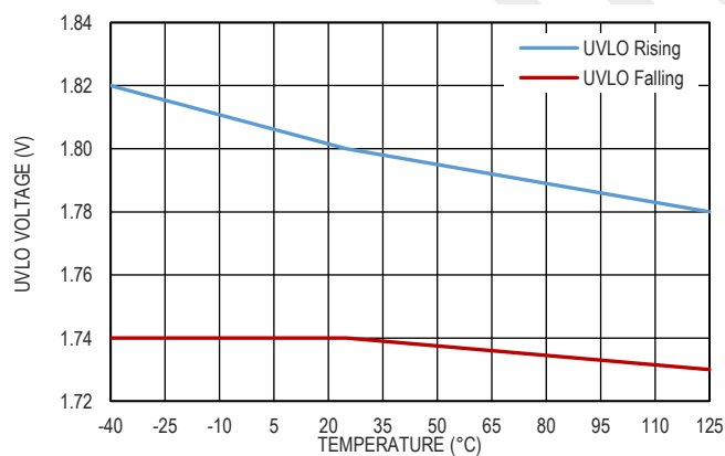
图 14. UVLO 阈值
