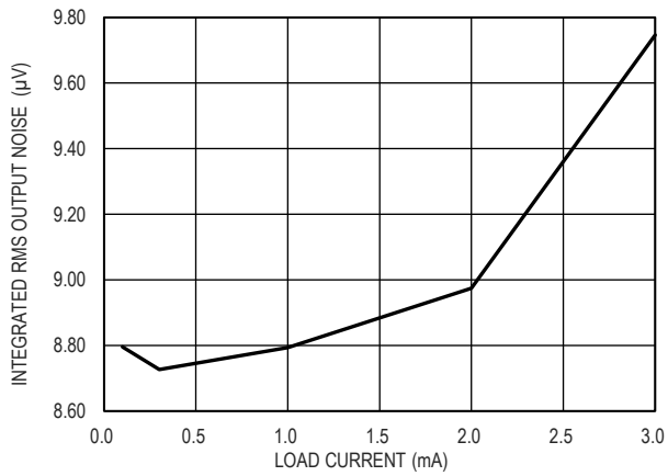
图 16. 积分 RMS 输出噪声, V_{IN}=5V , V_{OUT}=3.3V
