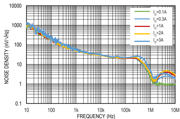
图 15. 输出噪声谱密度, V_{IN}=5V , V_{OUT}=3.3V
