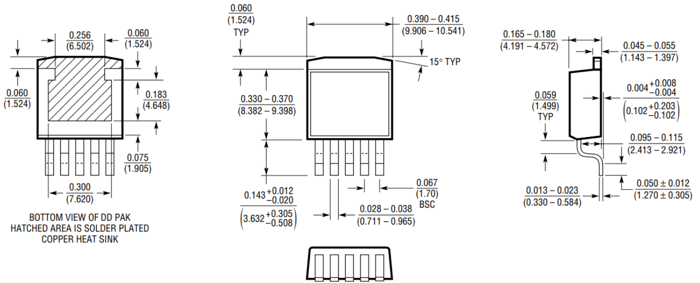
图 21.5 引脚 TO-263
