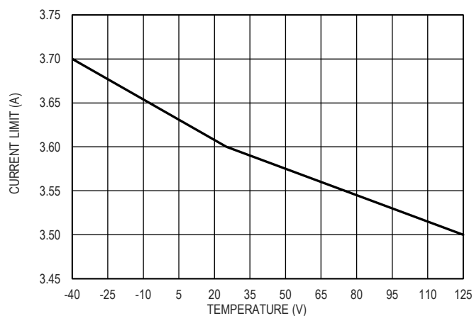
图 12. 输出限流值和温度的关系
