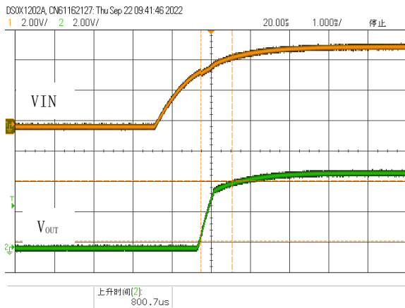
图 18. 软启动, V_{IN}=5.5V , V_{OUT}=5.0V , I_{OUT}=3A
