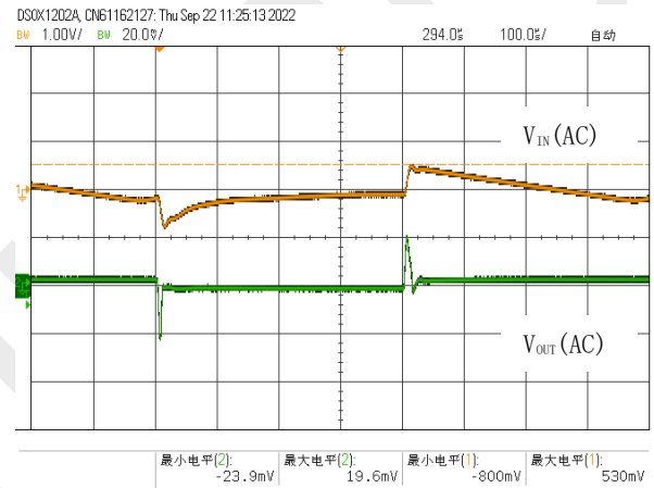
图 19. 负载瞬态响应, V_{IN}=2.8V , V_{OUT}=1.8V , I_{OUT}=300mA to 3A
