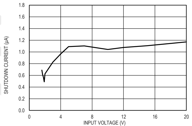
图 7. 关机电流和输入电压的关系
