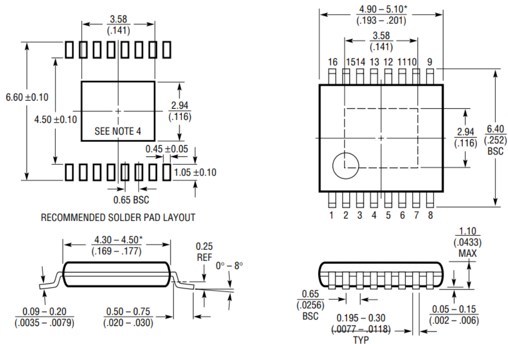
图 22.16 引脚 TSSOP
