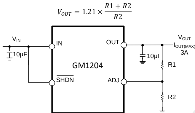
图 20. 由外部电阻决定的输出电压
