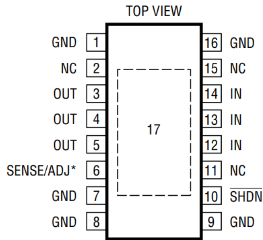
图 3 引脚配置
