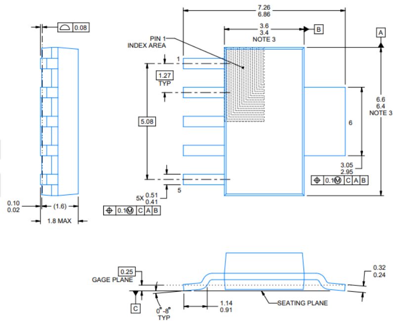
图 22.5 引脚 TO-263
