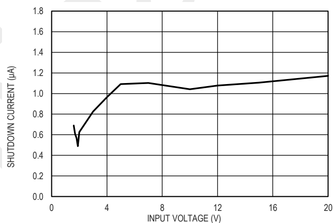
图 7. 关机电流和输入电压的关系
