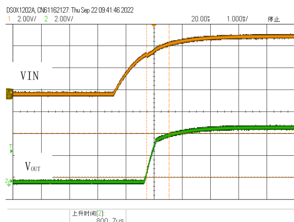
图 18. 软启动, V_{IN}=5.5V , V_{OUT}=5.0V , I_{OUT}=1.5A
