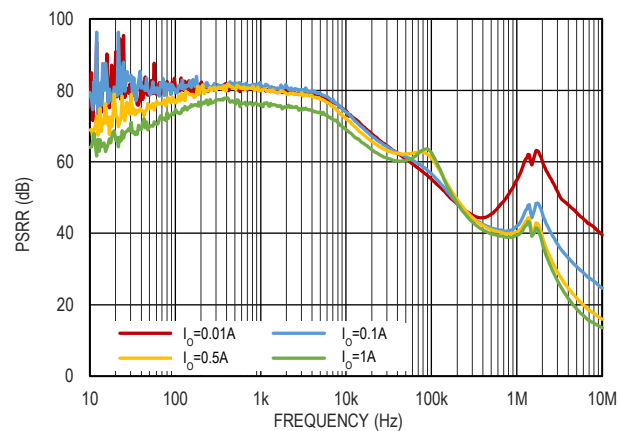
图 17. 电源电压纹波抑制比, V_{IN}=5V , V_{OUT}=3.3V
