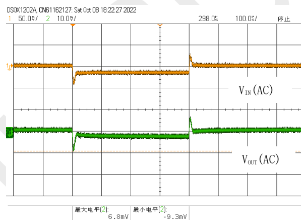
图 19. 负载瞬态响应, V_{IN}=2.8V , V_{OUT}=1.8V , I_{OUT}=100mA to 1.5A
