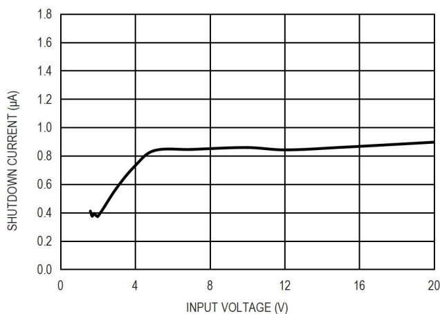
图 7. 关机电流和输入电压的关系
