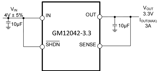
图 1 典型应用
