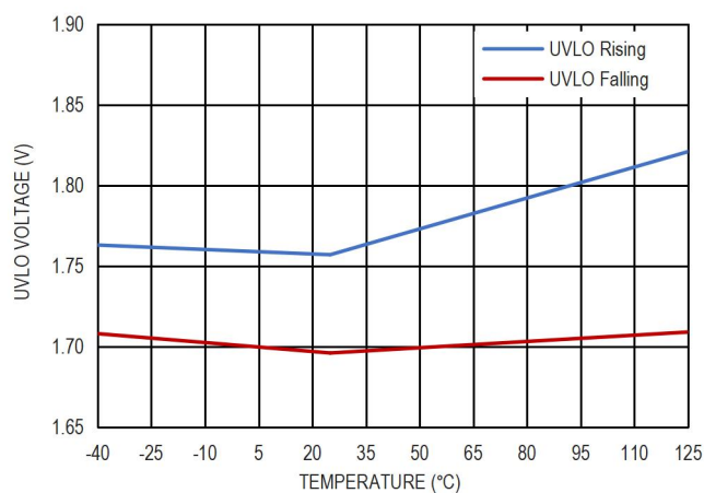
图 14. UVLO 阈值
