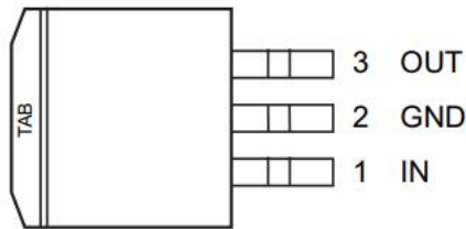
3 引脚 TO-263 裸露焊盘必须焊接到 PCB 上 图 2 引脚配置
