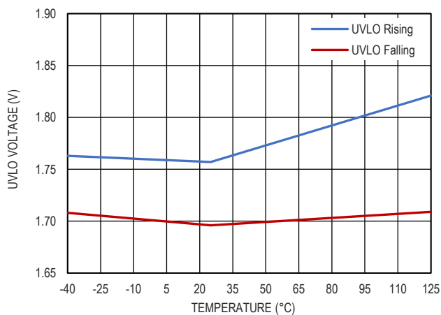
图 14. UVLO 阈值
