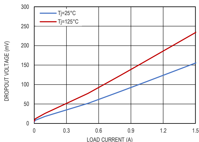
图 4. 压差电压和负载电流的关系
