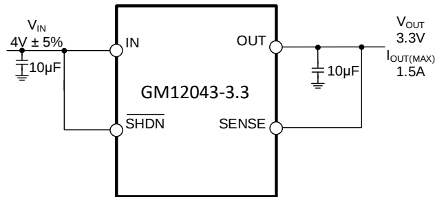
图 1 典型应用
