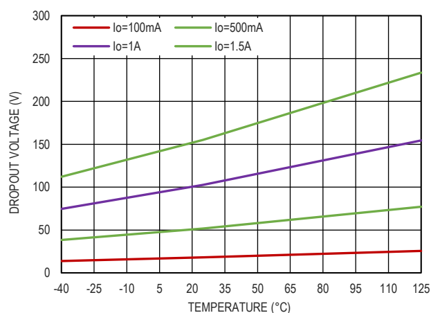
图 5. 压差电压和温度的关系
