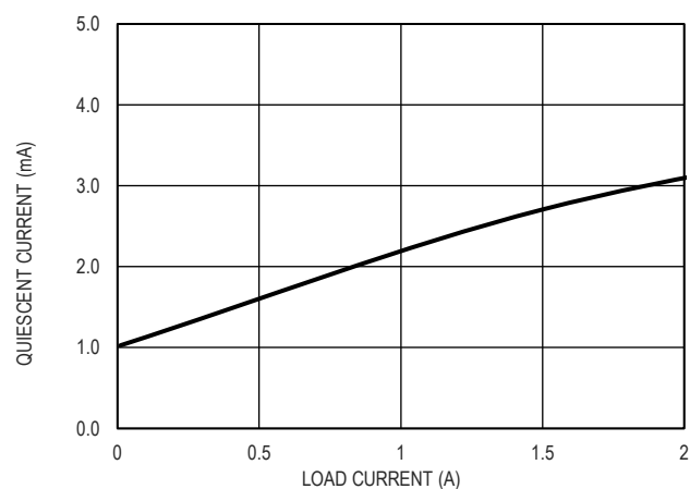
图 5. 静态电流和输入电压的关系, I_{OUT}=10mA
