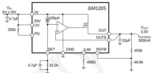
图 1 典型应用
