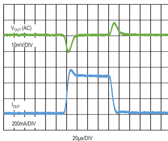
图 20. 负载瞬态响应, V_{IN}=4.3\text{V} , V_{OUT}=3.3\text{V} , I_{OUT}=1\text{mA} to 500\text{mA}
