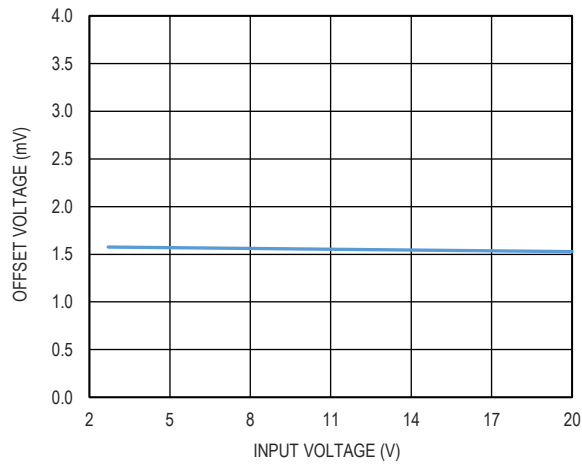
图 5. |V_{OUT} - V_{SET}| 和输入电压的关系, V_{OUT} = 1.5V
