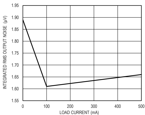
图 17. 积分 RMS 输出噪声, V_{IN}=5\text{V} , V_{OUT}=3.3\text{V}
