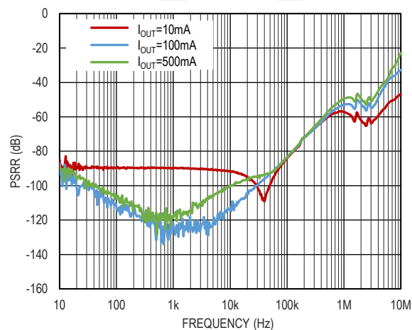
图 18. 电源电压纹波抑制比, V_{IN}=5\text{V} , V_{OUT}=3.3\text{V}
