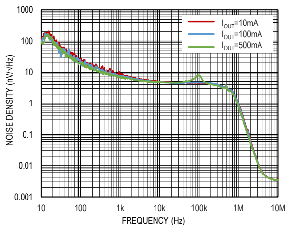
图 16. 输出噪声谱密度, V_{IN}=5\text{V} , V_{OUT}=3.3\text{V}
