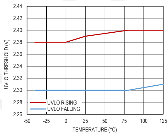
图 12. UVLO 阈值
