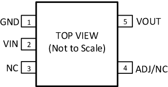
图 3. SOT-23 引脚配置(顶视图)
