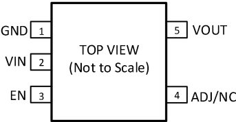
图 2. SOT-23 引脚配置(顶视图)
