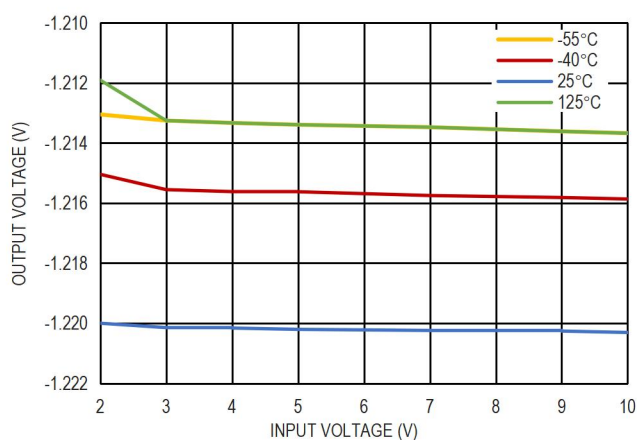
图 6. ADJ 引脚电压与 vs. 输入电压的关系
