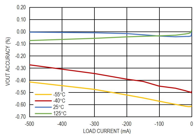
图 8. 固定输出电压 V_{OUT} 与负载电流的关系
