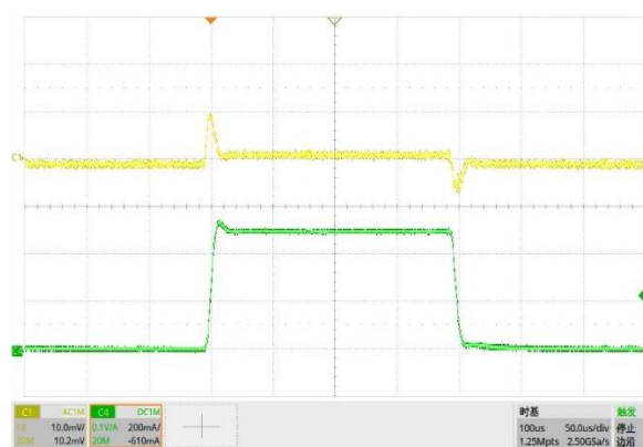
图 19. 负载瞬态响应, V_{OUT} = -5V , I_O = -10mA 至 -500mA
