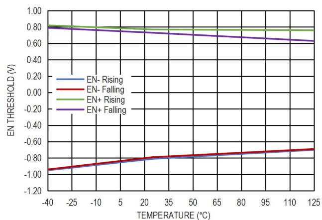
图 16. EN 阈值和结温的关系
