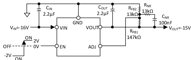
图 23. 更改可调输出 LDO 以降低噪声
