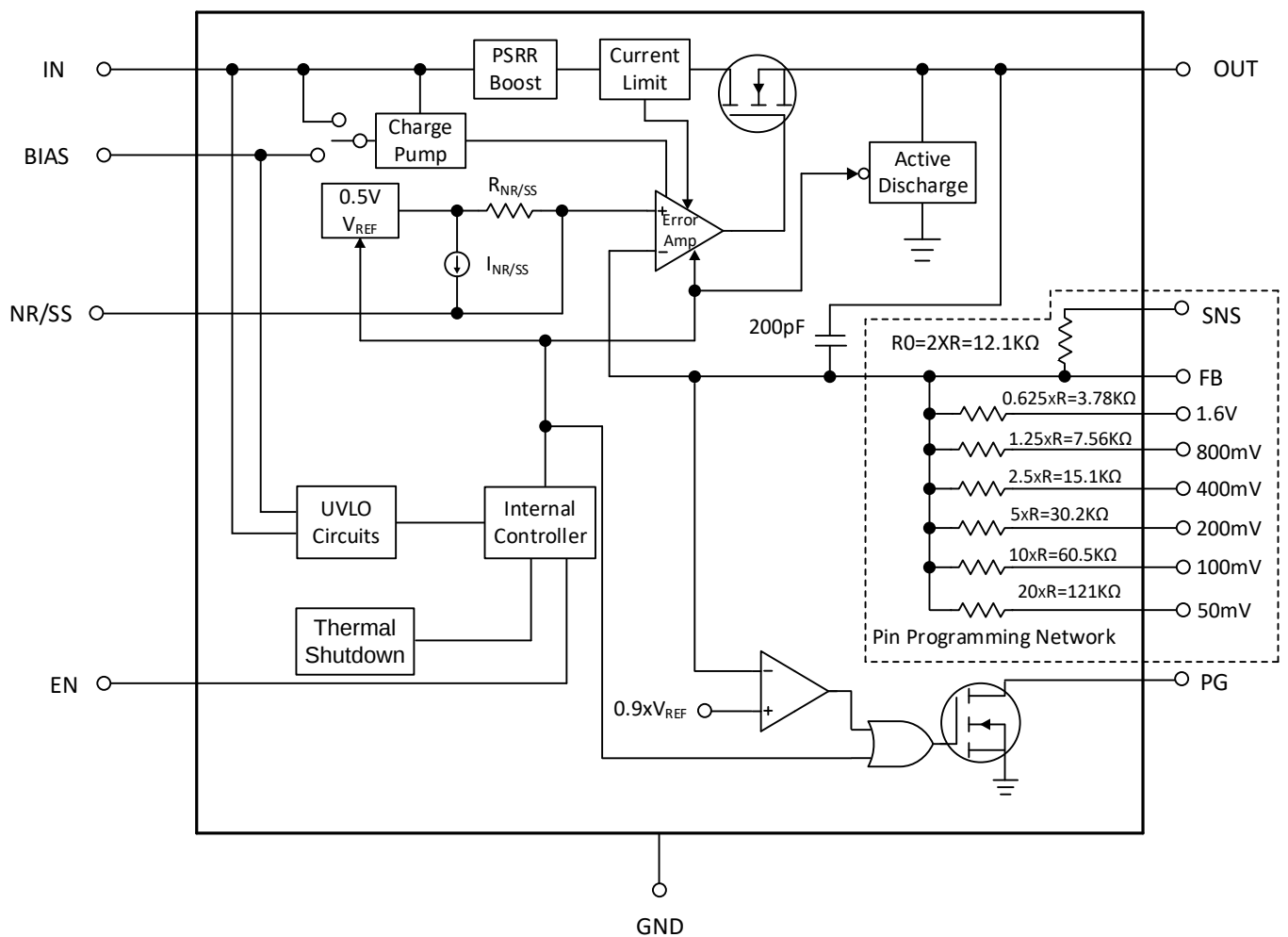
图 3. GM1503-1 方框图
