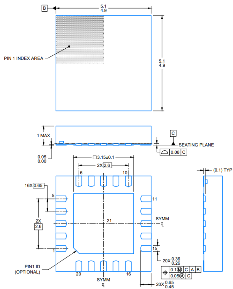
图 32. 20 引脚 QFN (5 毫米 x 5 毫米) 所有线性尺寸均以毫米为单位
