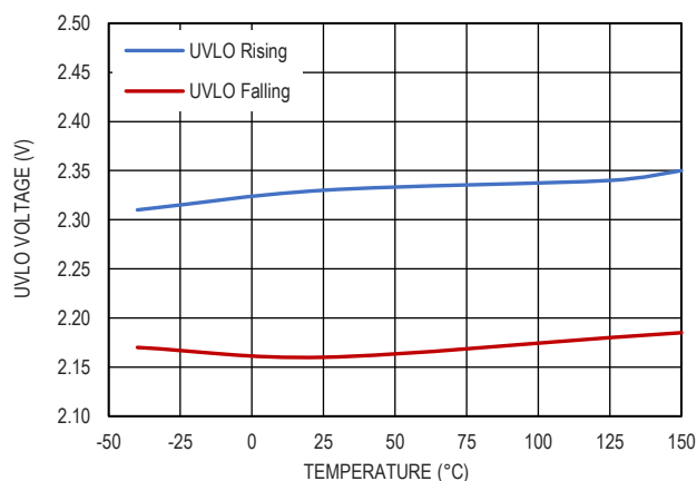
图 16. UVLO 阈值和温度的关系
