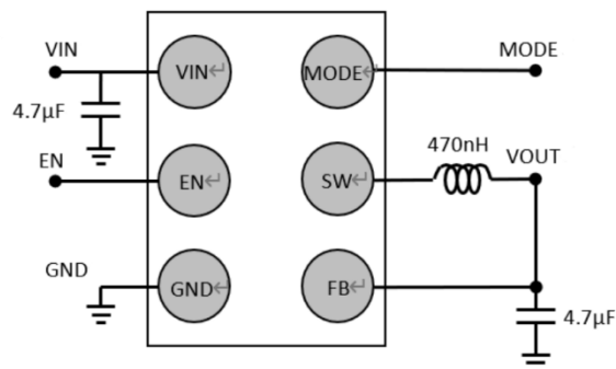
图1. 典型应用
