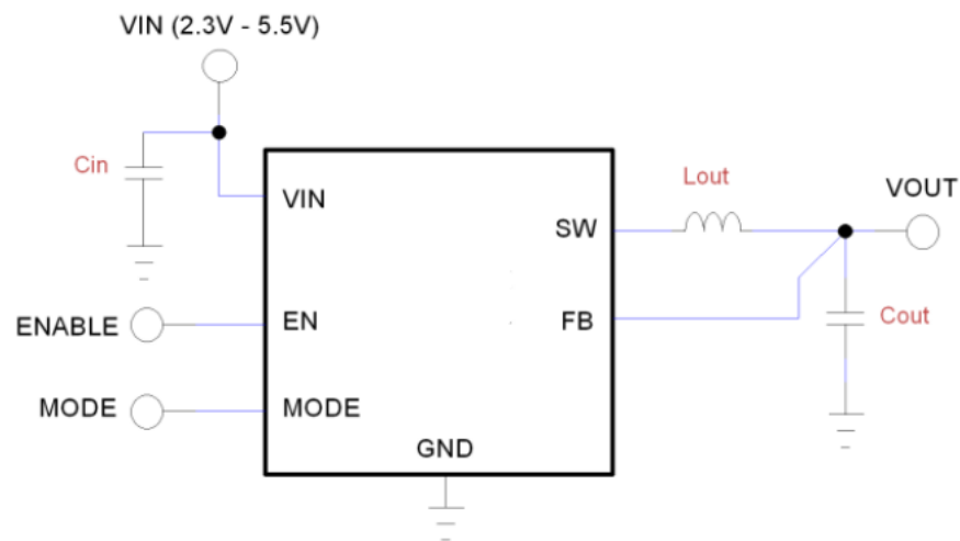
图 44. 应用电路
