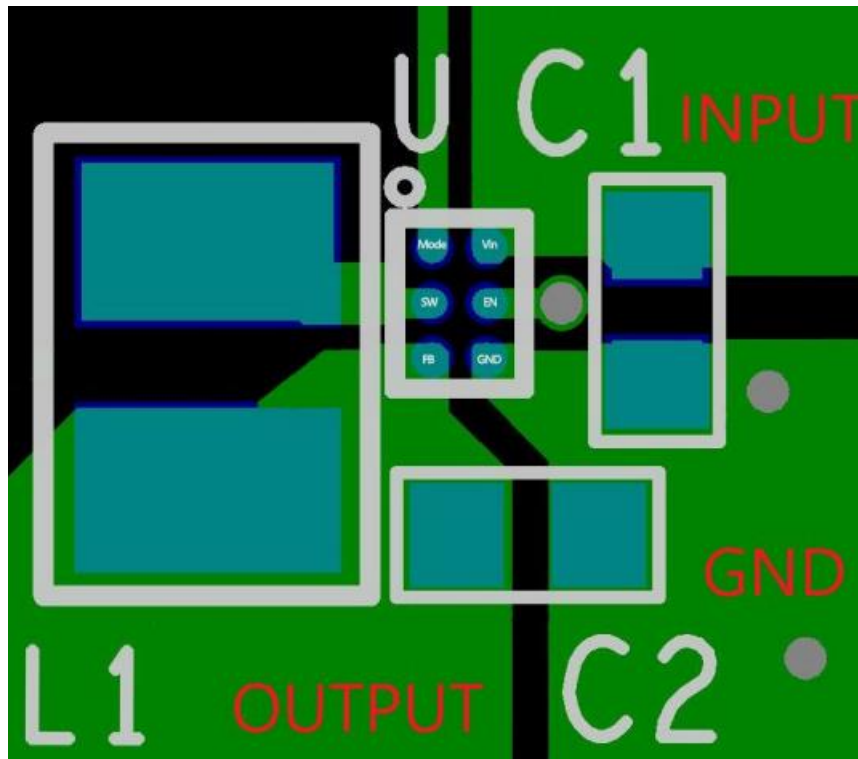
图 45. 顶层布局
