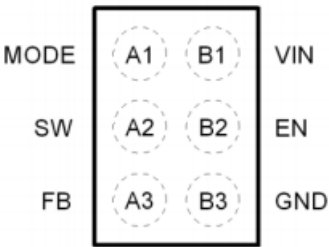
图 3. 顶视图
