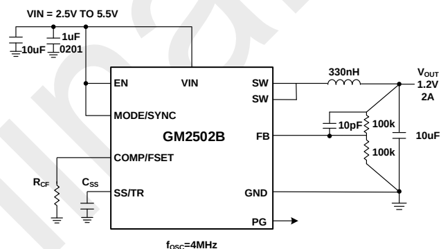
图 2. 4MHz 典型应用
