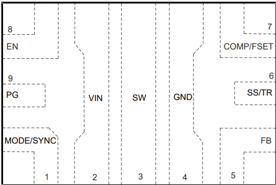
9 引脚 LQFN 图 4 引脚配置
