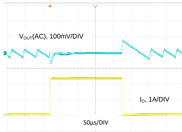
图 24. V_{OUT} = 1.2V , I_O = 0.1A 至 2.5A , 低功耗模式
