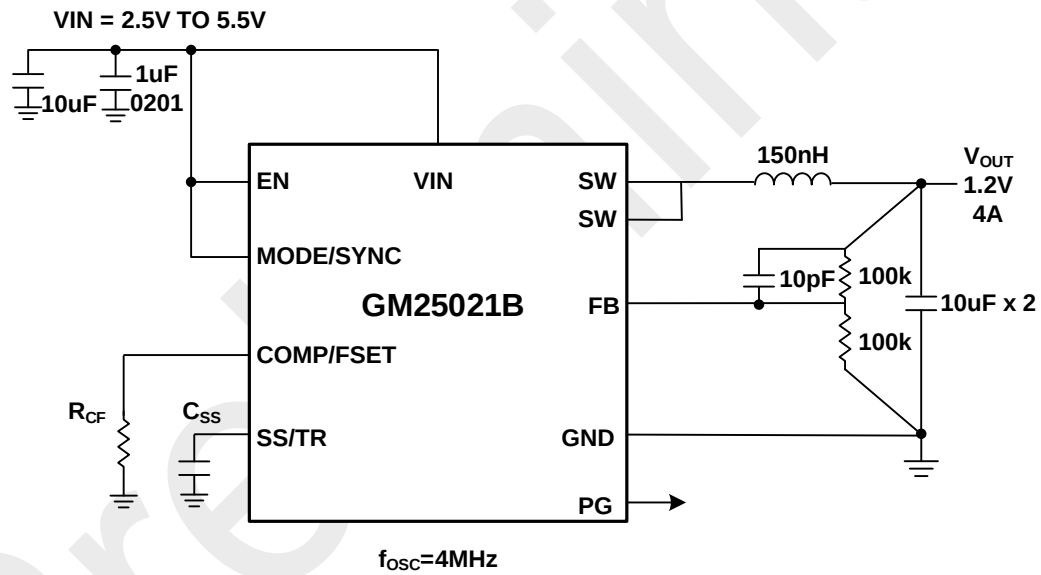
图 30. 4MHz, V_{IN}=3.3\text{V} , V_{OUT}=1.2\text{V} , I_{LOAD}=4\text{A}
