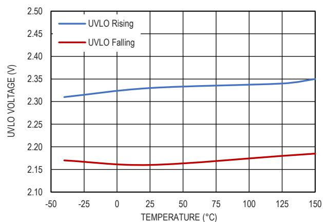
图 16. UVLO 阈值和温度的关系
