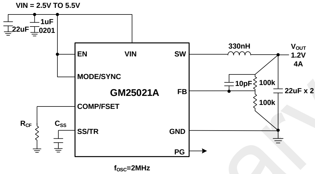
图 29. 2MHz, V_{IN}=3.3\text{V} , V_{OUT}=1.2\text{V} , I_{LOAD}=4\text{A}
