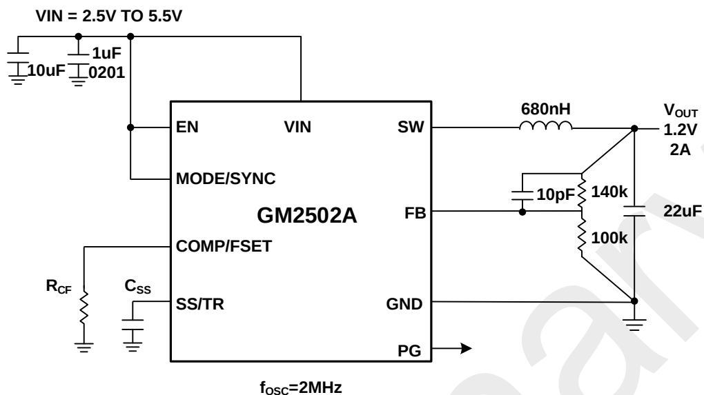
图 27. 2MHz, V_{IN}=3.3V , V_{OUT}=1.2V , I_{LOAD}=2A
