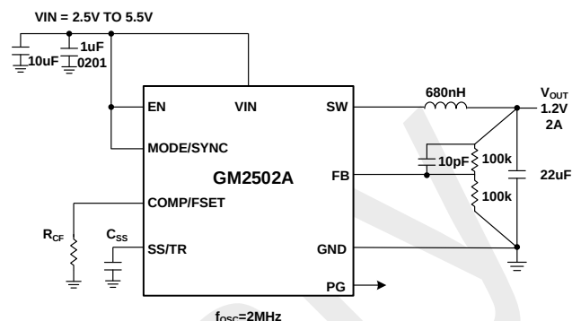
图 1. 2MHz 典型应用
