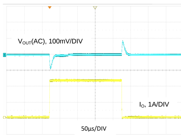
图 22. V_{OUT} = 1.2V , I_O = 0.1A 至 2.5A , FPWM 模式
