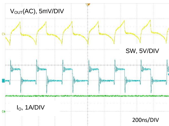
图 14. V_{OUT} = 1.2\text{V} , I_O = 1\text{A} , FPWM 模式
