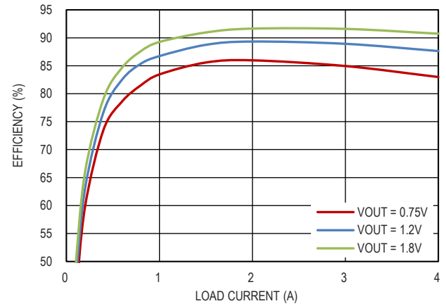
图 5. 效率曲线, V_{IN} = 5V , 低功耗模式
