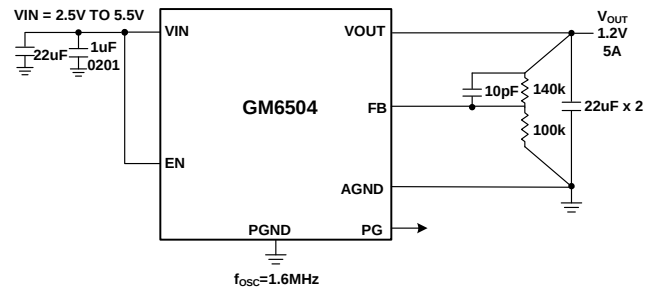
图 1. GM6504 典型应用
